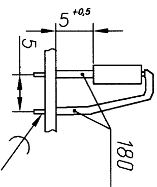
Установка ХР2,ХР5,ХР8
