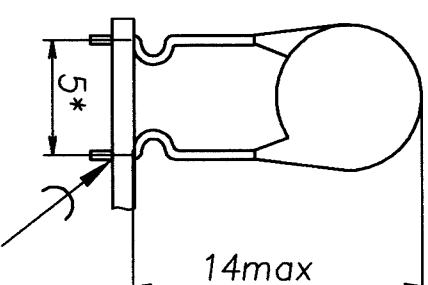
Установка R74
